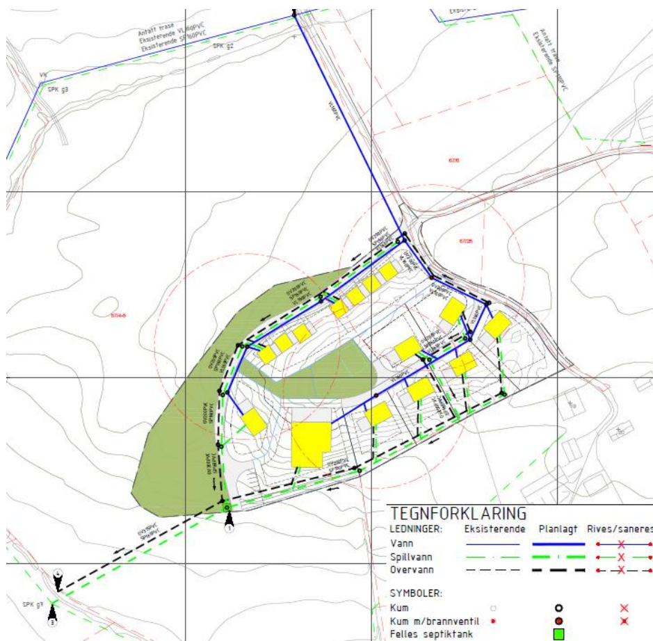
Figur 16 Kartusnitt fra vedlagt VA-plan
