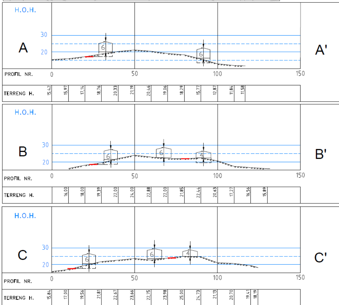
Figur 14 Tverrsnitt som viser planlagte byggehøyders samsvar med eksisterende terreng. Modellen baserer seg på variant 1
